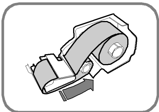
Рисунок 1.14 – Протяжка ленты
