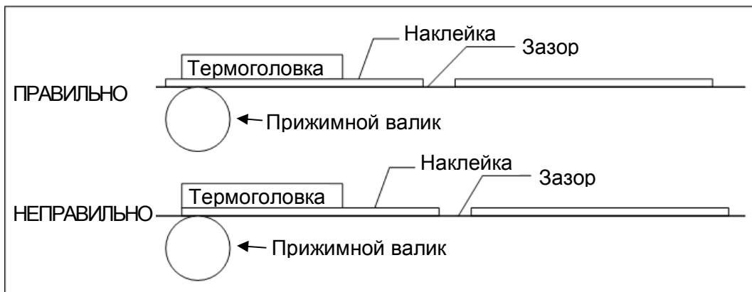
Рисунок 1.18 – Варианты правильного и неправильного положения ленты этикеток
